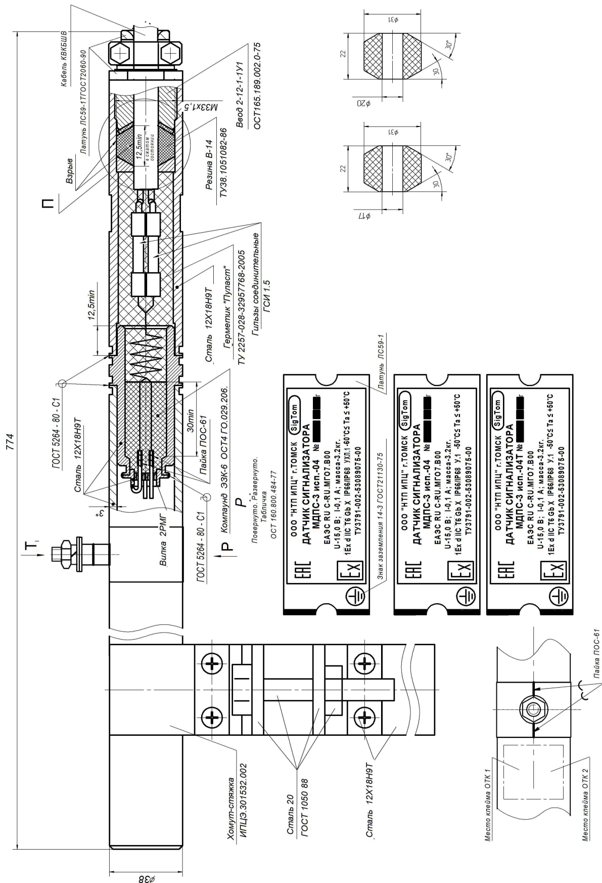
Рисунок 16 – Чертёж средств взрывозащиты сигнализатора МДПС-3 исп. 04.
