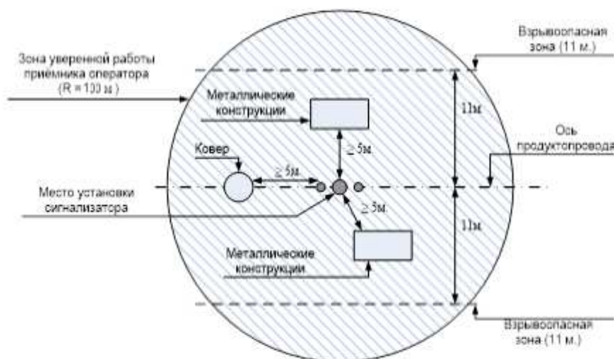
Рисунок 7 – Схема установки переносного сигнализатора «РЕПЕР-3В» относительно коверов и других металлических конструкций.
