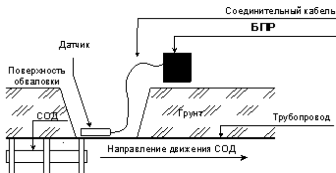
Рисунок 8 – Схема установки переносного сигнализатора «РЕПЕР-3В» исполнения «МДПС-3Р».
