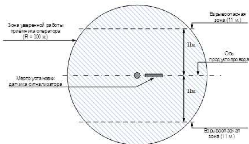
Рисунок 10 – Схема установки переносного сигнализатора «РЕПЕР-3В» исполнения «МДПС-3Р» относительно коверов и других металлических конструкций.
