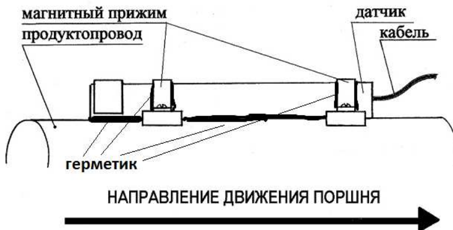
Рисунок 9 – Схема установки переносного сигнализатора исполнения «МДПС-ЗР» с акустическим каналом.
